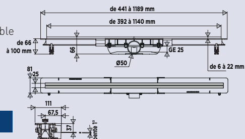
hauteur du profilé réglable de 6 à 22 mm: s'adapte à l'épaisseur du carrelage
